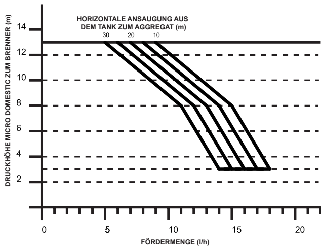
VERTIKALE ANSAUGUNG AUS DEM TANK ZUM AGGREGAT 2,5 m
